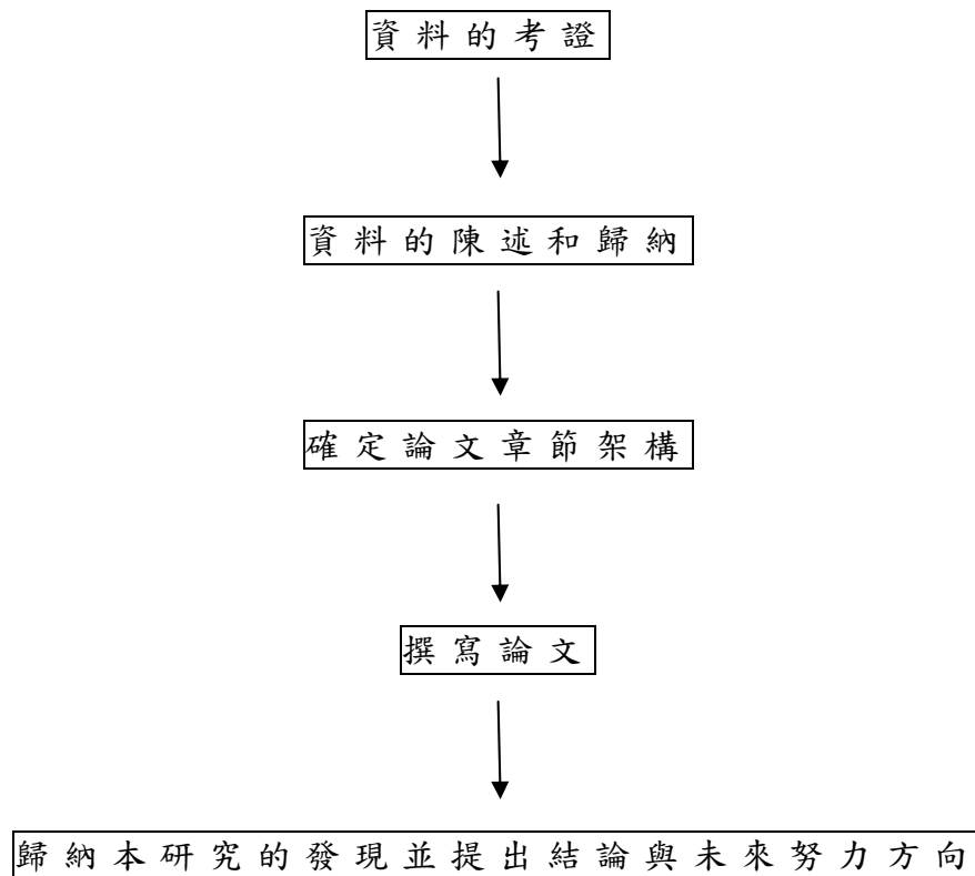
圖 1 研究流程圖
