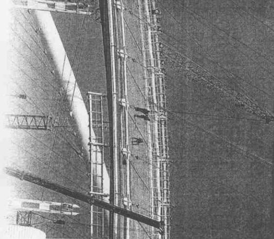
▲施工人員在田徑場及開閉會場的頂端穿樓施工，身影在重型機械及吊車的襯托下格外渺小。特派記者侯永全／攝與傳真
