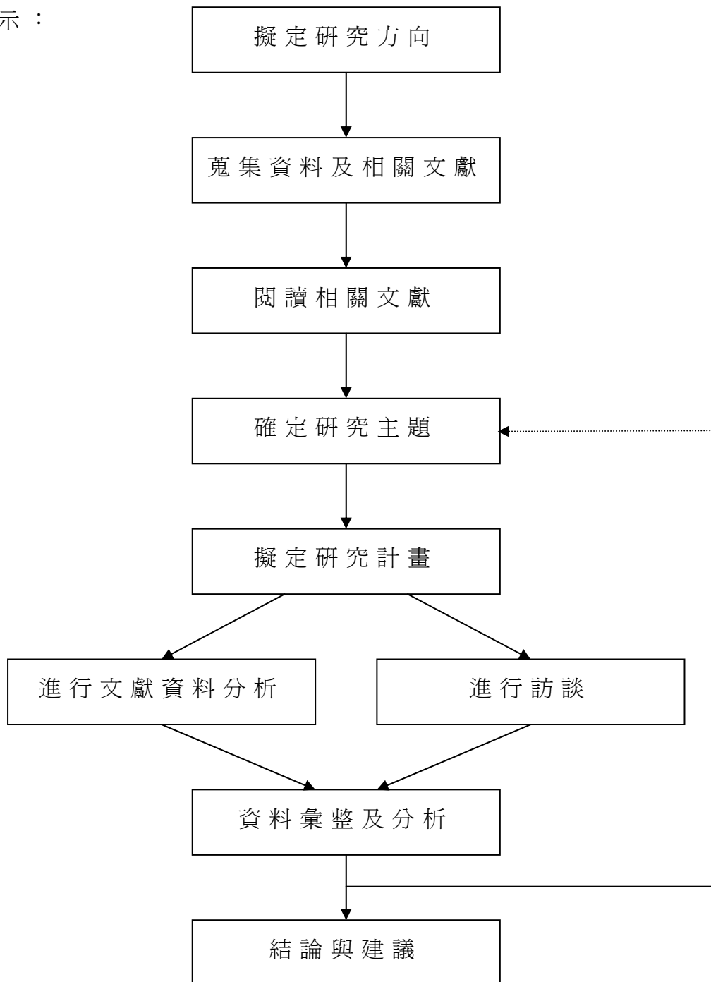
圖 1：研究流程圖
